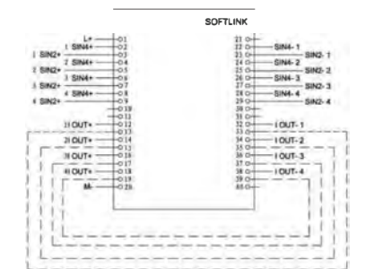
300 ISO-4C
