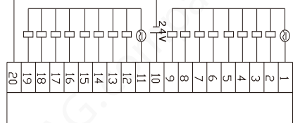
300 322-1HH01
